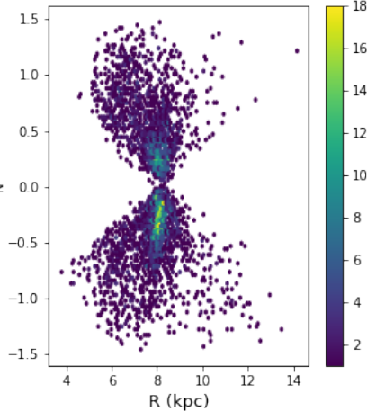
Galah DR3
