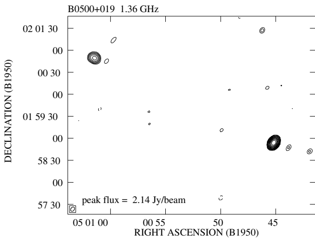
Fig. 5. 0500+019 at 1.36 GHz.
