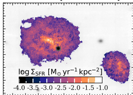
SFR2: 20 \text{ Myr} < t \leq 570 \text{ Myr}
