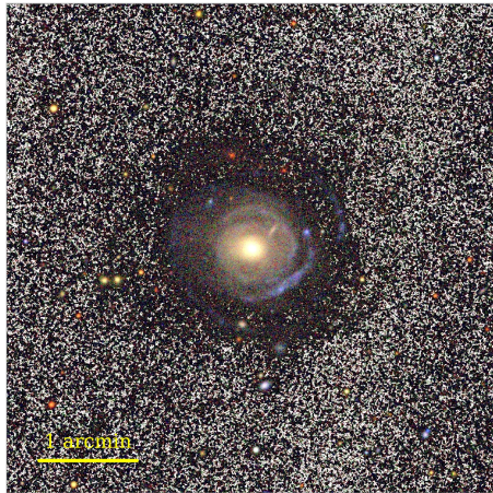
SDSS
