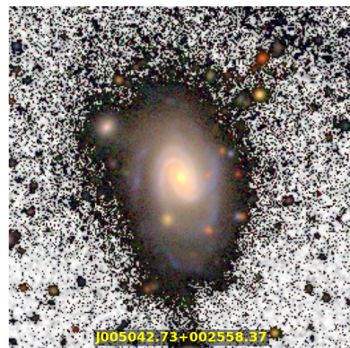
\log(M_*/M_\odot) = 10.6
