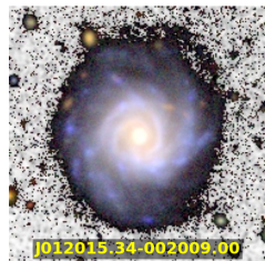
\log(M_*/M_\odot) = 10.6
