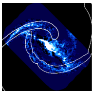
NGC 2566
