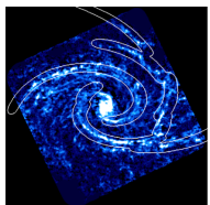
NGC 2997
