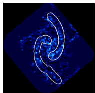
NGC 2283
