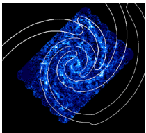
NGC 628
