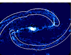
NGC 1300
