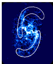
NGC 1385
