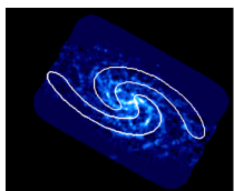
IC 1954
