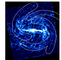
NGC 5643
