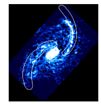
NGC 5248
