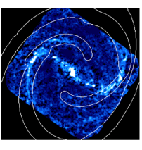
NGC 4548
