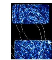
NGC 6744
