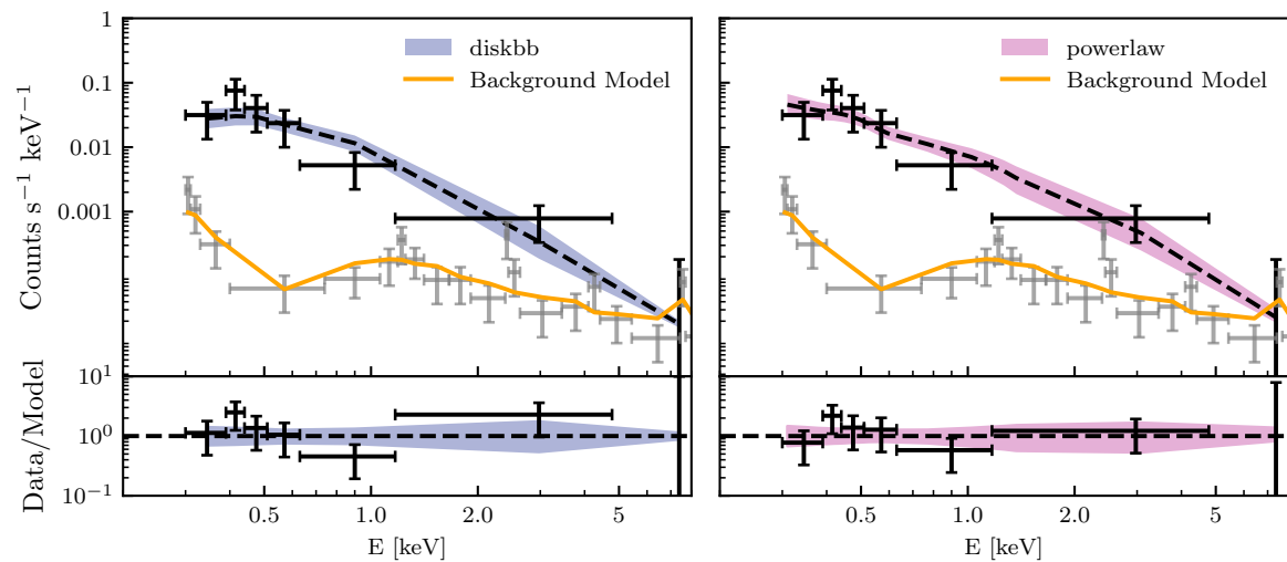
Swift-XRT4
