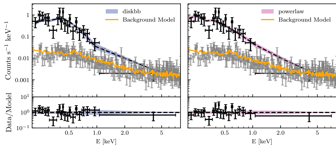
Swift-XRT3
