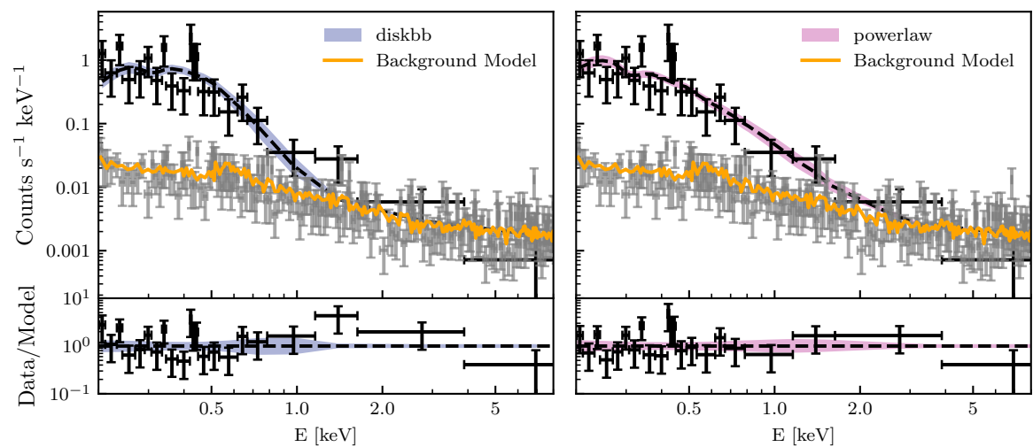
eRASS3
