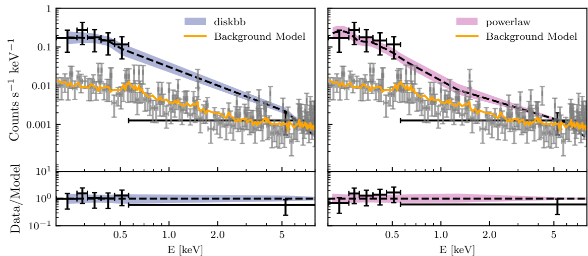
eRASS4
