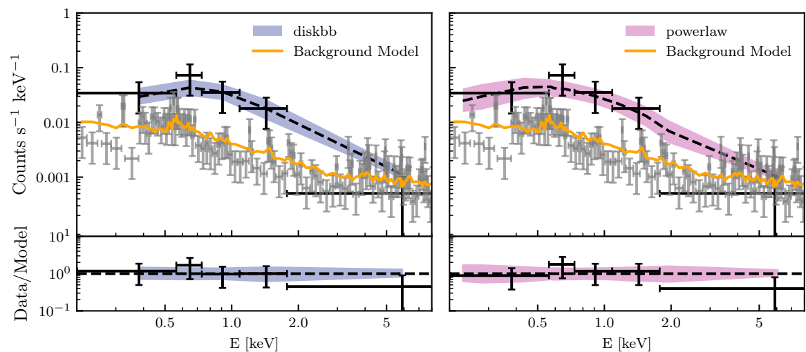
eRASS4
