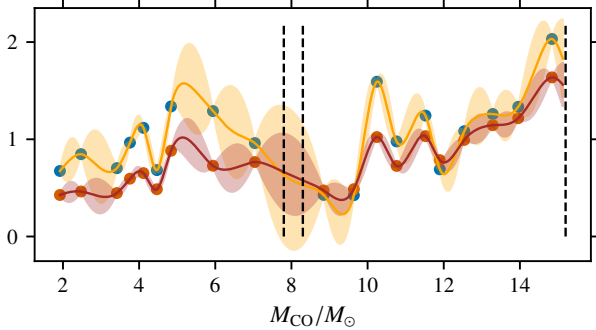
Z = Z_{\odot} , Case B1
