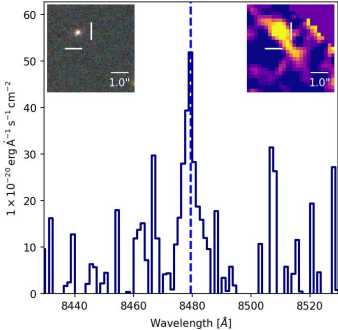
z = 5.975 LyA 43.1a
