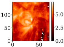
Radiance - Ne VIII 770 Å AR 12958
