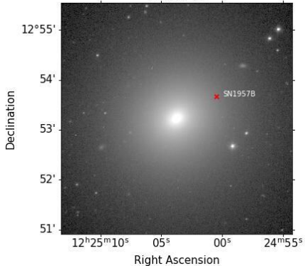
Messier 84
