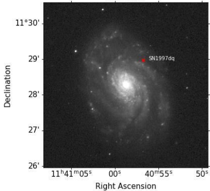
NGC 3810
