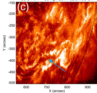
SDO AIA 05-Apr-2011 06:17:56 UT
