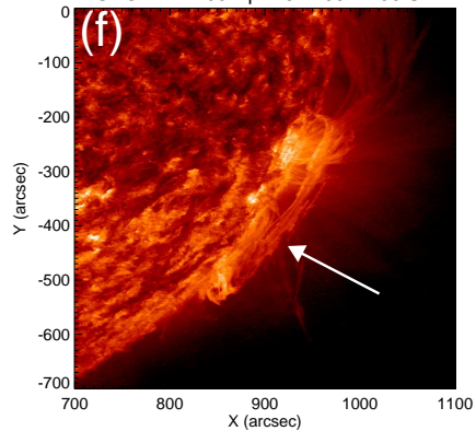
SDO AIA 05-Apr-2011 06:17:56 UT
