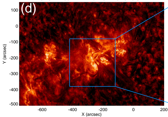
SDO AIA 304 27-Mar-2011 13:28:20 UT
