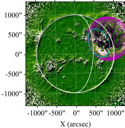
b. STA/EUVI 195 Å 11:30:00 UT
