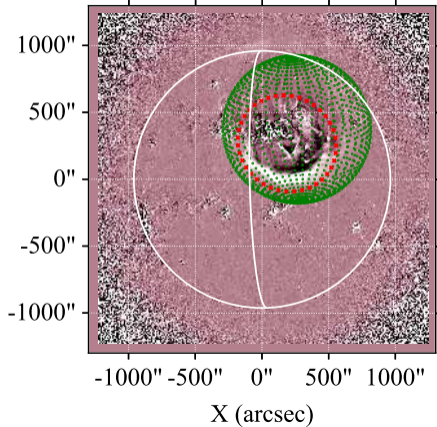
a. SDO/AIA 211 Å 11:29:57 UT
