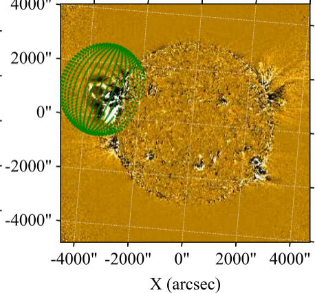
c. SoI/O/EUI 174 Å 11:20:50 UT
