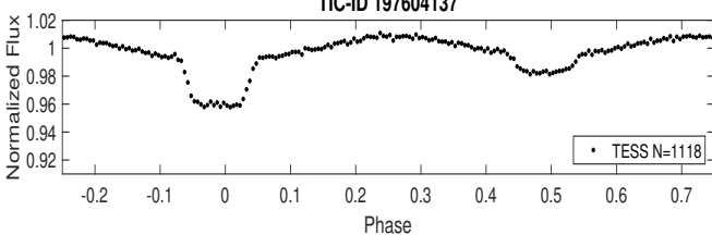
Gaia-ID 6637219674994191744
