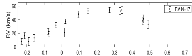
Gaia-ID 2048990809445098112
