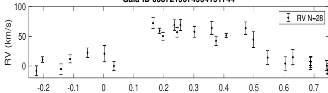
Gaia-ID 6637219674994191744
