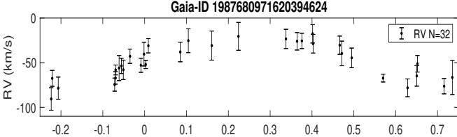
Gaia-ID 1987680971620394624
