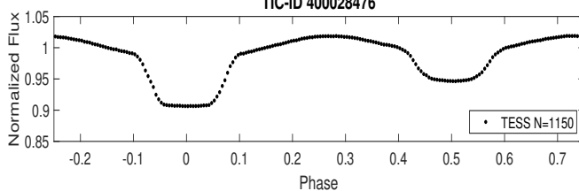
Gaia-ID 2048990809445098112
