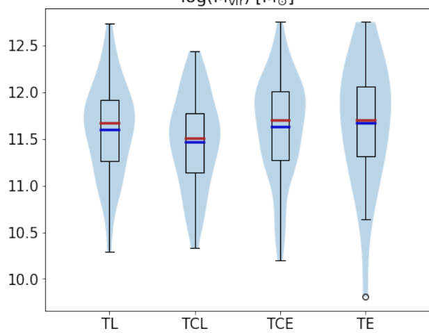
\log(M_{vir}) [M_{\odot}]
