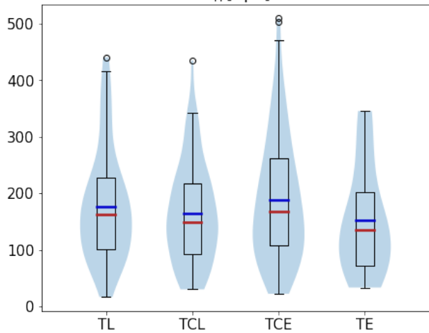
H_0 t_c
