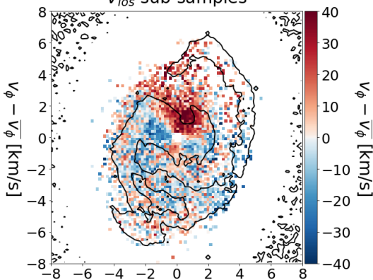
V_{los} sub-samples
