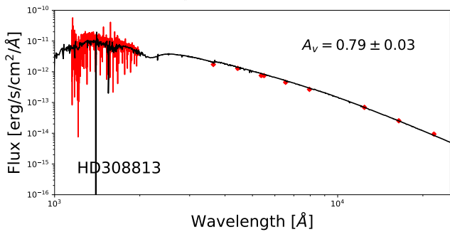
(l) HD 308813
