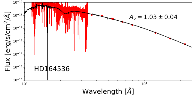
(v) HD 164536
