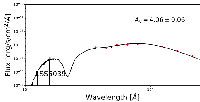
(o) LS 5039
