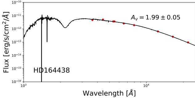
(u) HD 164438
