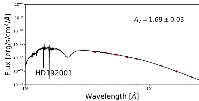
(z) HD 192001
