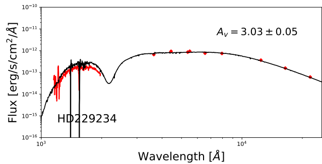
(i) HD 229234
