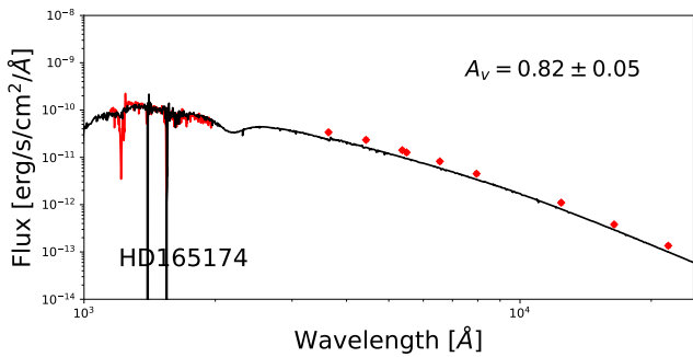
(w) HD 165174
