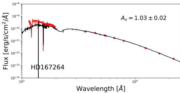
(y) HD 167264
