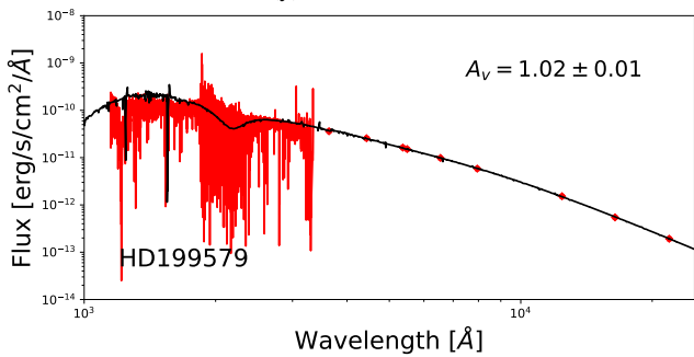
(j) HD 199579
