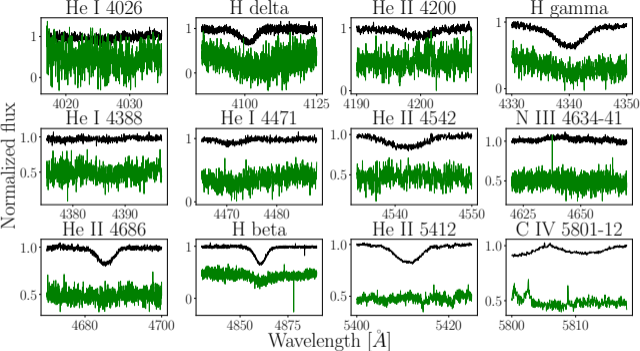
(q) V747 Cep
