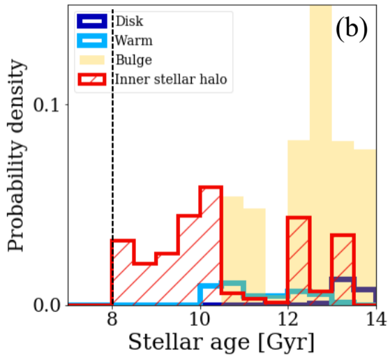
NGC 1427
