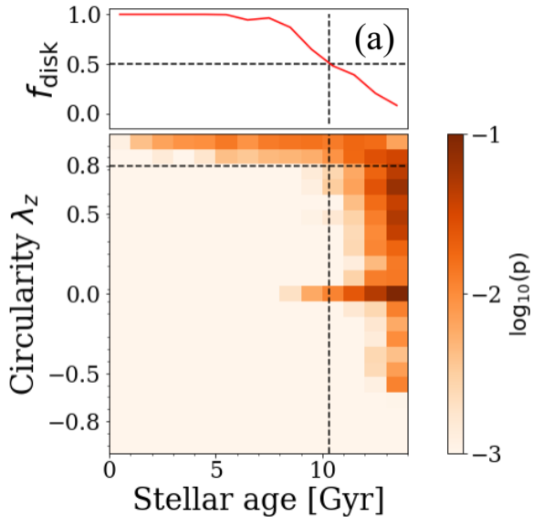
NGC 1380
