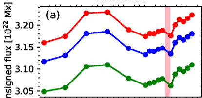
AR 11158
