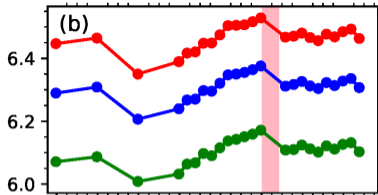
AR 11429
