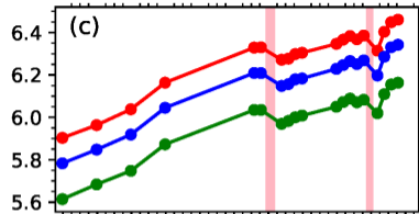
AR 12673
