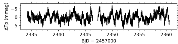
\delta Lup (s038)
