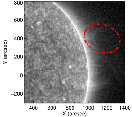
EUVI-A 171Å 13-April-2020 22:09 UT
