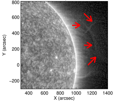
EUVI-A 171Å 13-April-2020 14:09 UT
