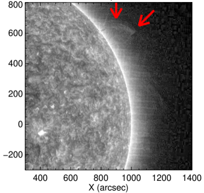
EUVI-A 171Å 12-April-2020 02:09 UT
