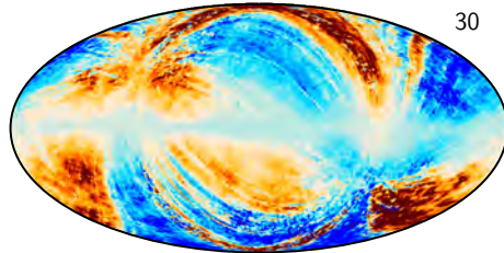
\frac{2018-2015-\Delta M-\Delta D}{2015-CMB}
