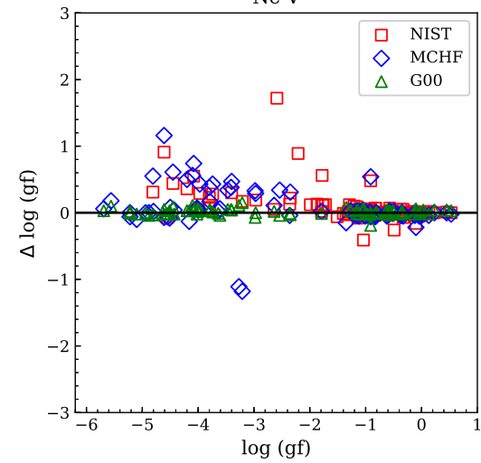
Ne V
