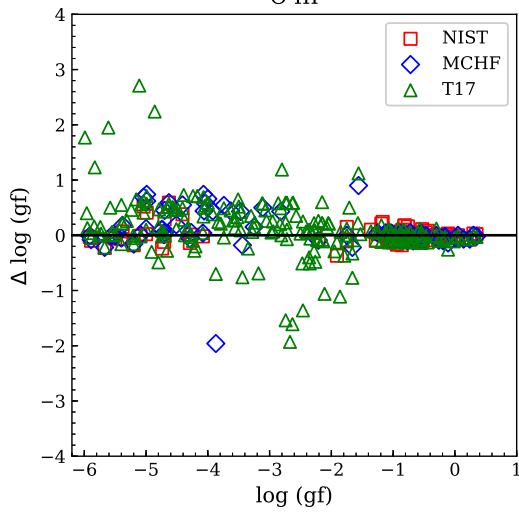
O III
