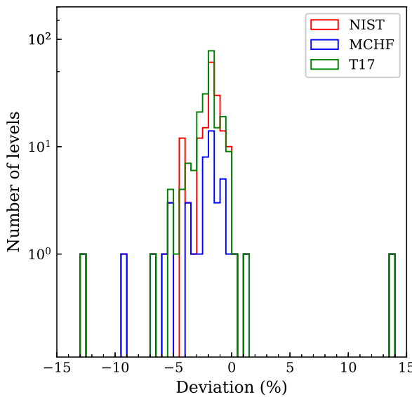
O III
