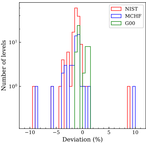
Ne V
