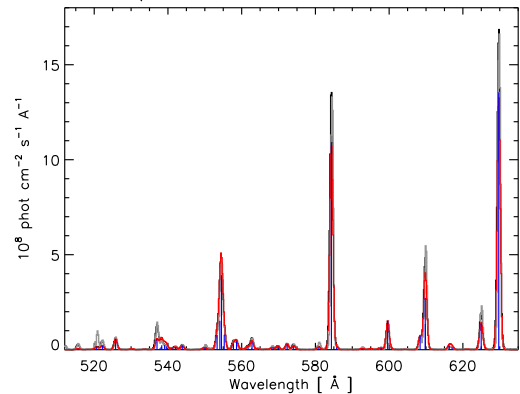
Quiet Sun PEVE + EVE + CHIANTI
