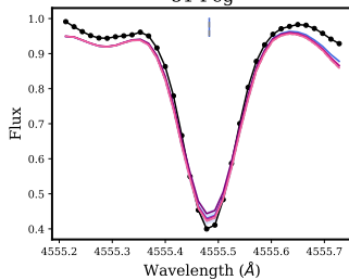
51 Peg
