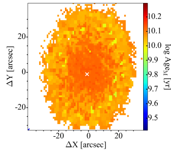
CALIFA/STECKMAP
