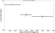
WFM (2-50 keV)
