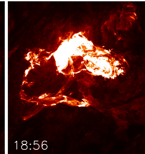
Evolution of 1-Jan-2014 flare
