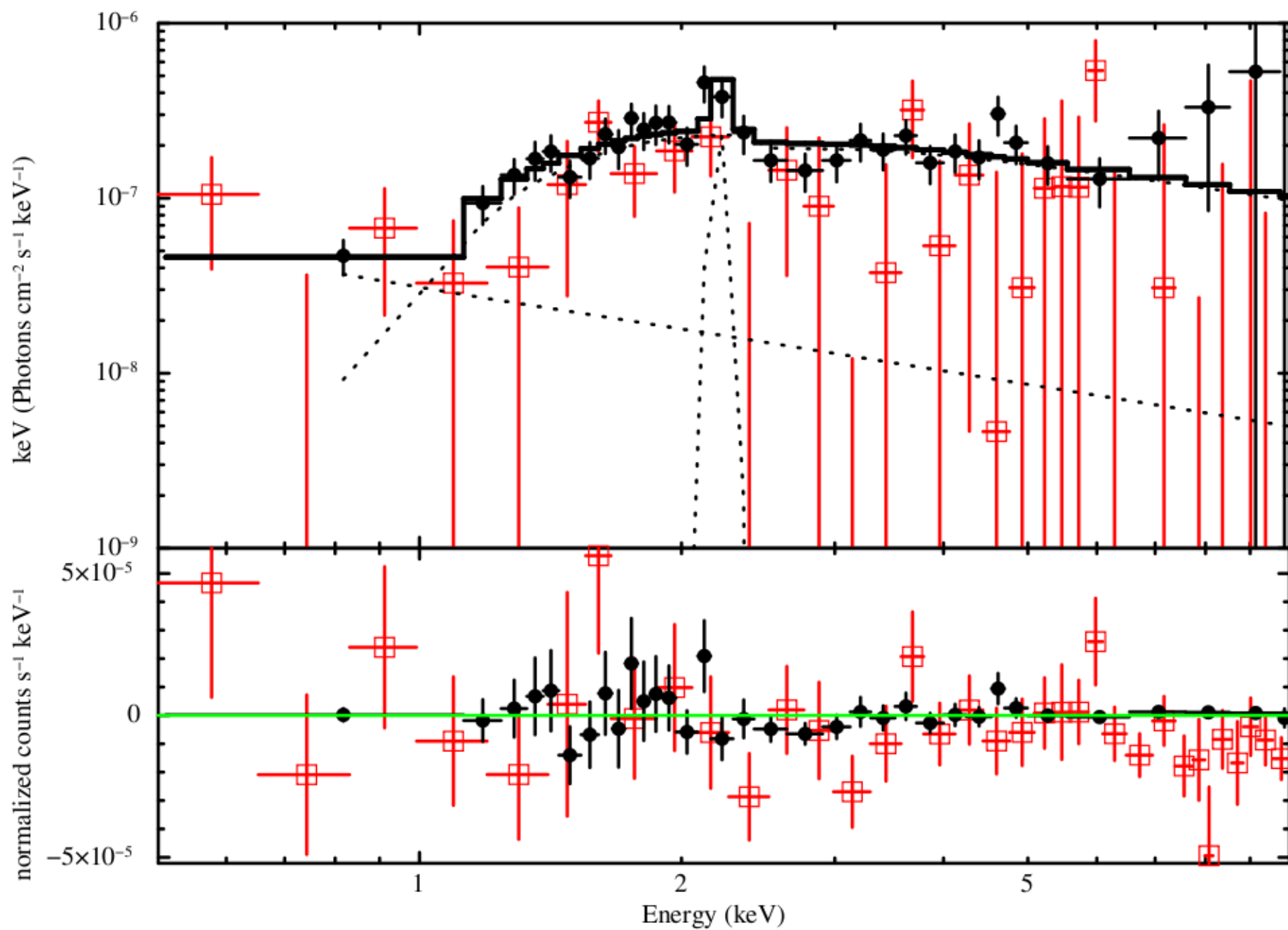
SRC 307 - z=1.90
