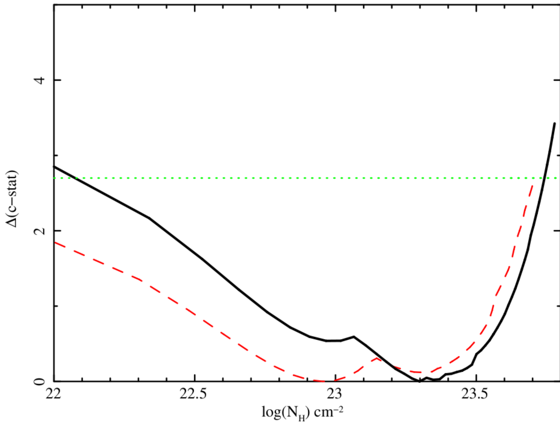
SRC 293 - z=3.88
