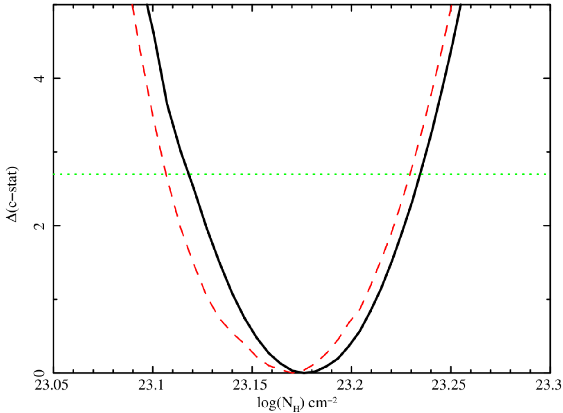
SRC 232 - z=2.291
