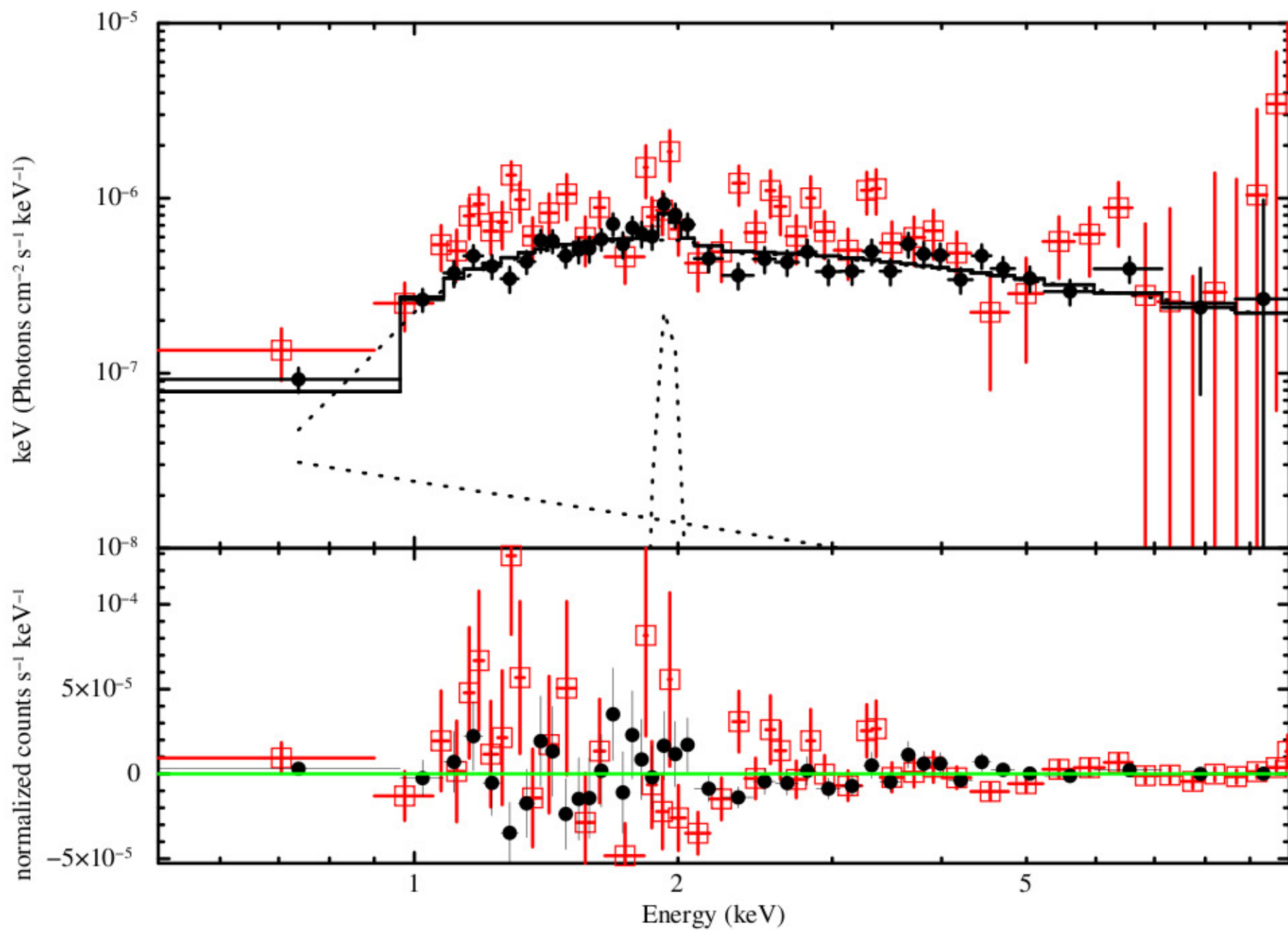
SRC 232 - z=2.291
