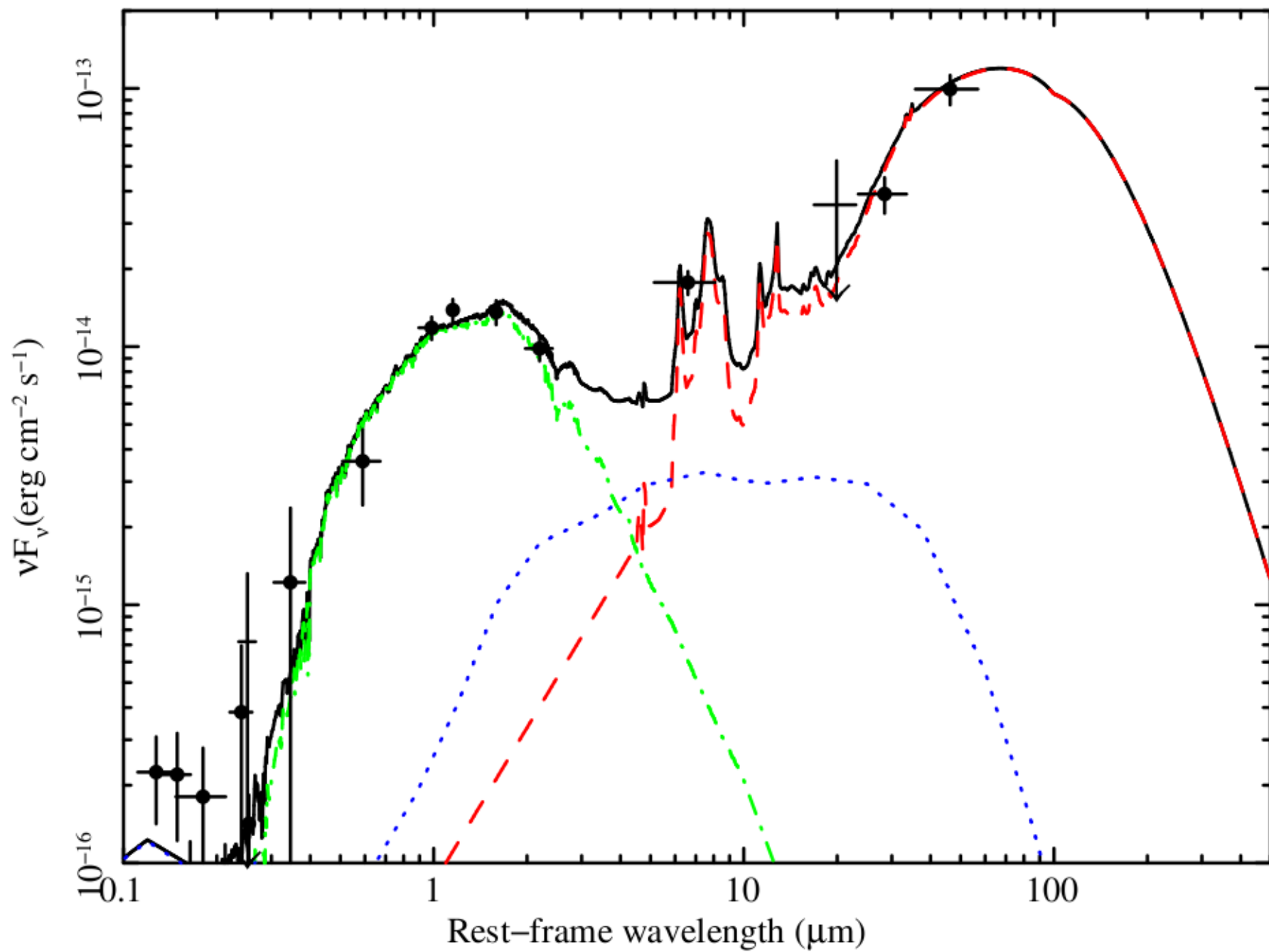
SRC 230 - z=2.61
