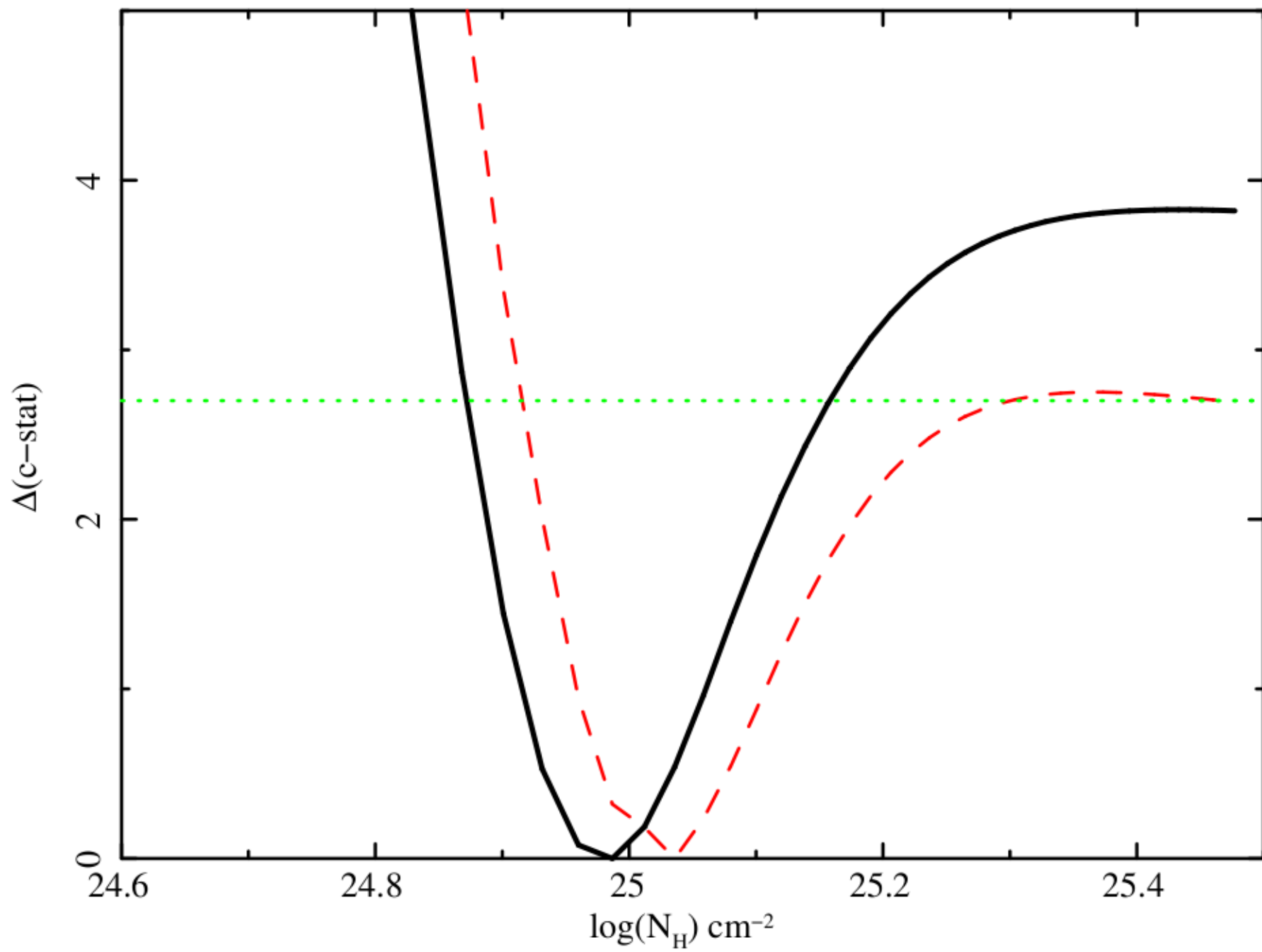
SRC 230 - z=2.61
