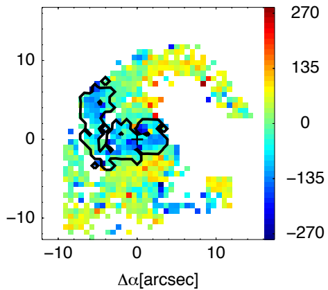
V_{NaD}
